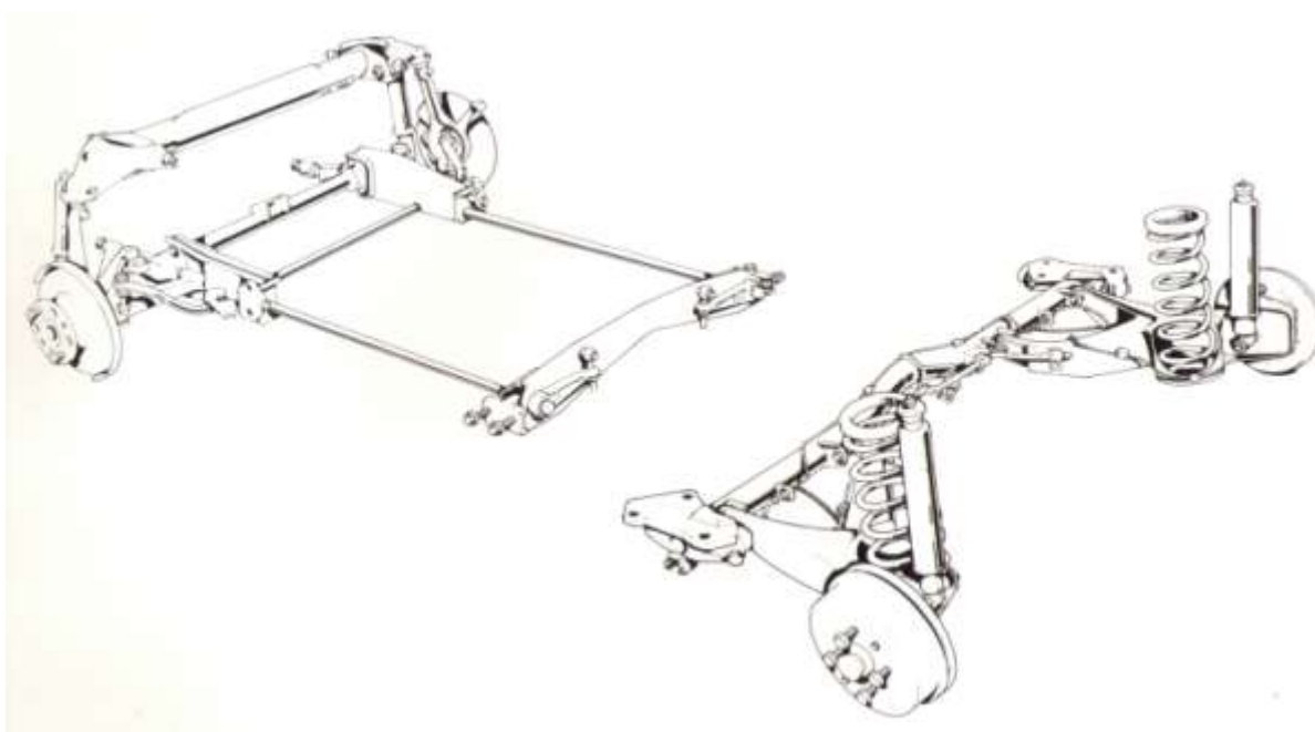
Abb. 4: Simca 1307 Fahrwerk / Aufhängung [Werkbild]
