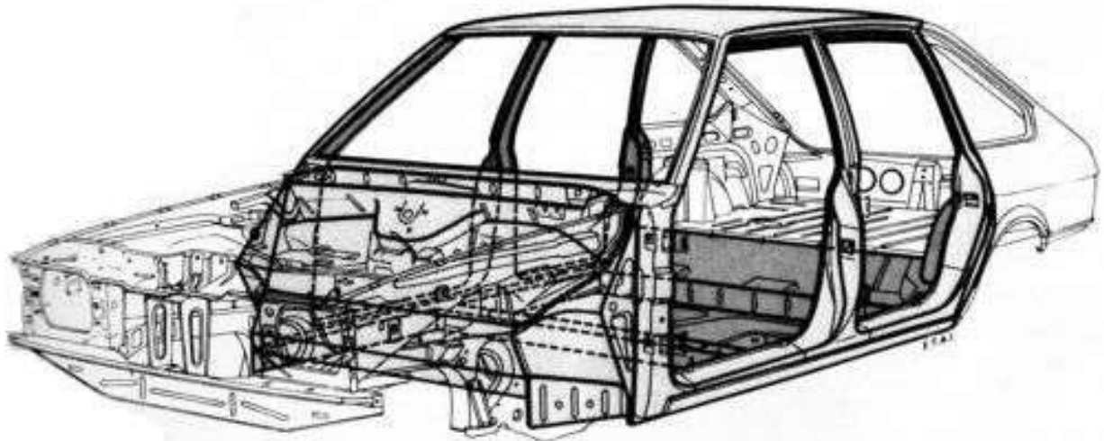
Abb. 2: Simca 1307 Karosserie in Explosionsdarstellung [Werkbild, ETAI]
