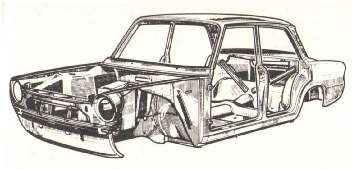
Abb. 2: Simca 1300 Rohkarosserie [Werkfoto]
