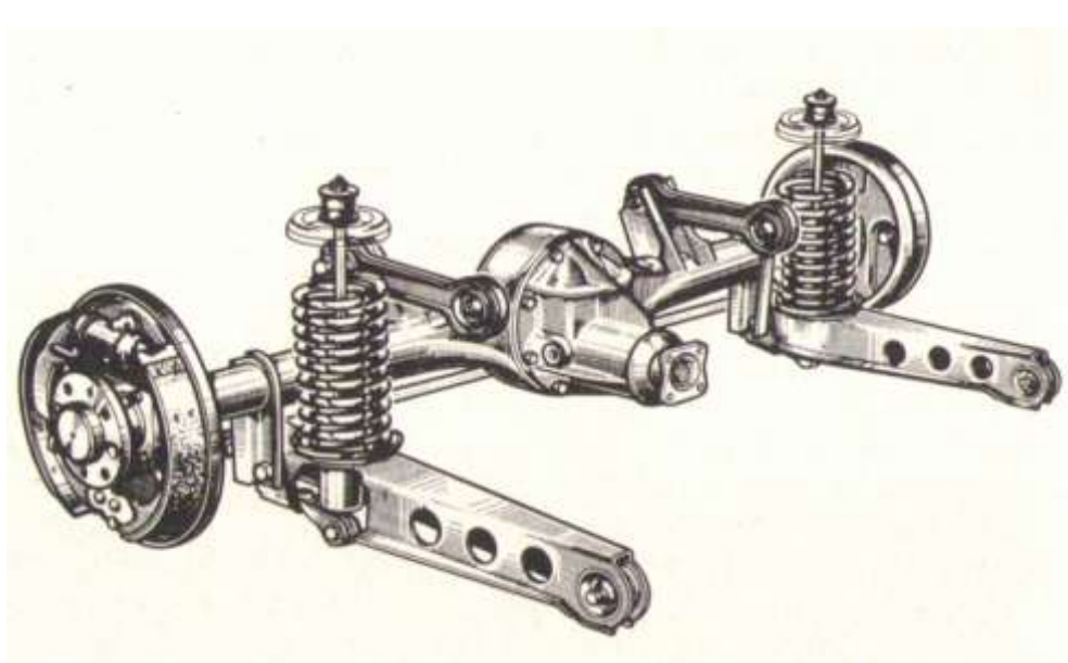
Abb. 4: Simca 1300 Hinterachse [Werkfoto]
