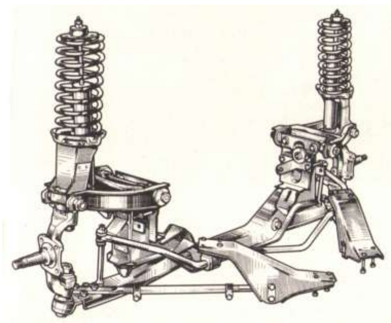
Abb. 3: Simca 1300 Vorderachse [Werkfoto]
