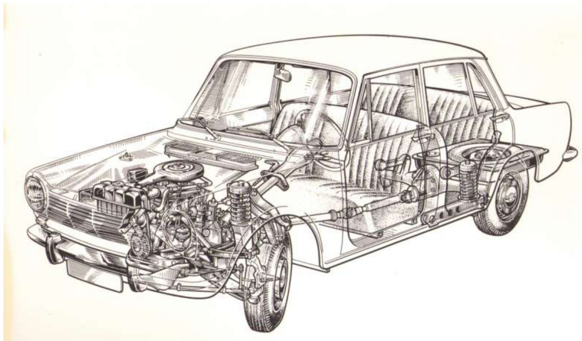
Abb. 1: Simca 1300 Röntgenblick [Werkfoto / ETAI]
